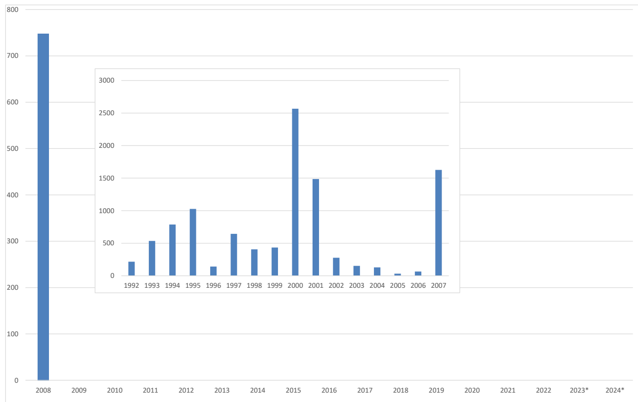
Rubéola, nº de casos por ano , Estado de São Paulo, 1992-2023*
